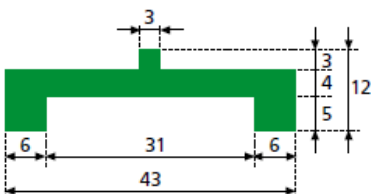
Profilo T rinforzato
